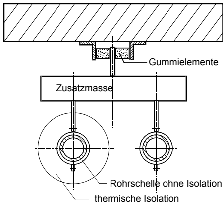
Abb. 15 Körperschalldämmung bei Kältemittelleitungen für erhöhte Schallschutzanforderungen.
