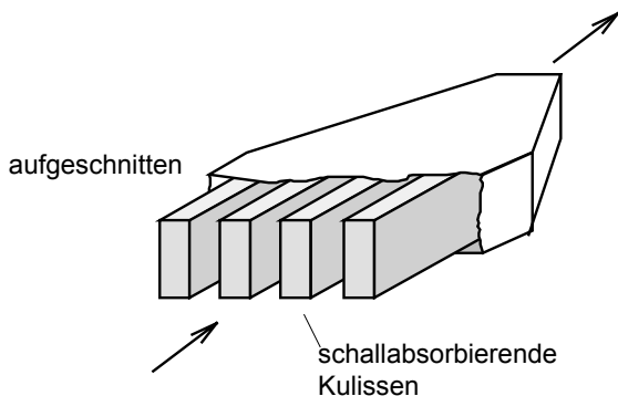
Abb. 6b Kulissenschalldämpfer (einseitig aufgeschnitten)
