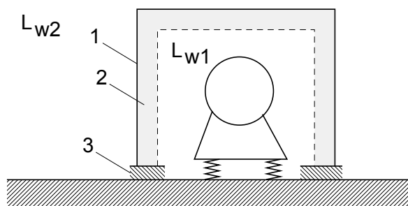
Abb. 5 Kapsel (1 Kapselwand, 2 schallabsorbierende Innenverkleidung, 3 körperschall-dämmende, dichte Auflage)
