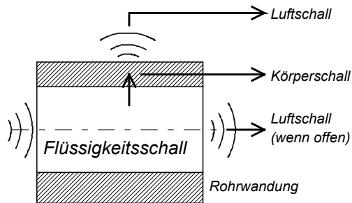
Abb. 4 Übertragungswege und Umwandlungen von Flüssigkeitsschall
