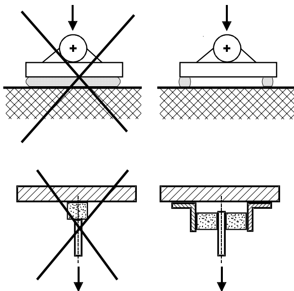
Abb. 9 Richtige Anwendung von Gummi
