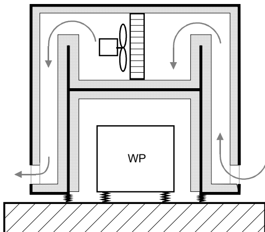
Abb. 16 Schematisch dargestellte Lärmschutzmassnahmen an einer aussen aufgestellten Luft/Wasser-Wärmepumpen.
