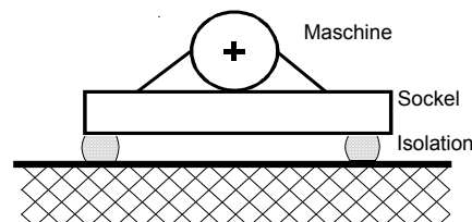
Abb. 10 Punktweise Lagerung einer Maschine (Einfachisolation)
