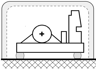
Abb. 17 Schematisch dargestellte Lärmschutzmassnahmen an einer innen aufgestellten Sole/Wasser oder Wasser/Wasser-Wärmepumpe.
