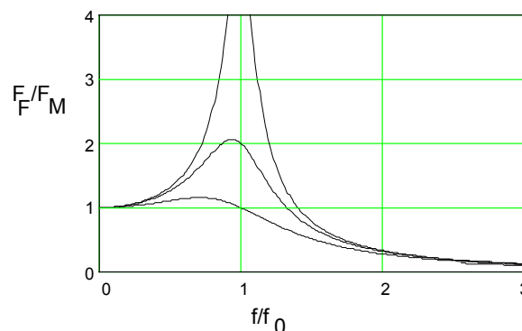
Abb. 8 Verhältnis F_F/F_M für verschiedene Dämpfungen (Reibung) in Funktion zur normierten Frequenz f/f_0 . f ist die Erregerfrequenz und f_0 die Resonanzfrequenz des Feder-Masse-Schwingers.
