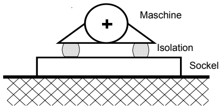
Abb. 13 Diese Anwendung eines Sockels ist nur bei leichten Geschosstrennedecken sinnvoll.
