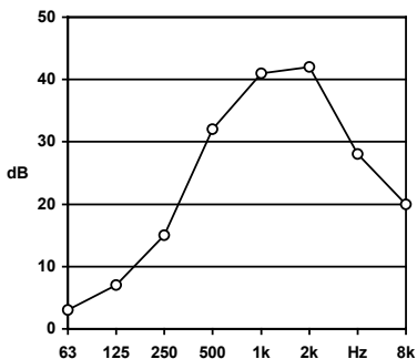
Abb. 8 Beispiel der Durchgangsdämpfung eines Absorptions-Schalldämpfers
