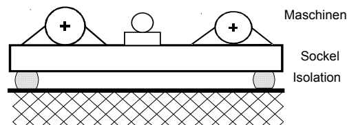
Abb. 12 Gruppe von Maschinen auf dem gleichen Sockel
