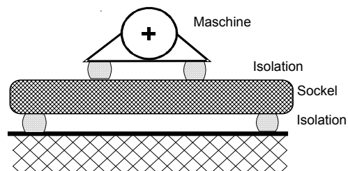
Abb. 11 Doppelisolation einer Maschine auf einer Geschosstrenndecke.
